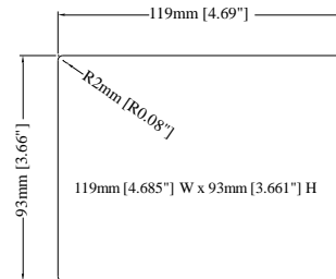
Cutout Dimensions
