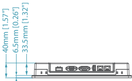
底視圖
