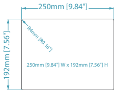
開孔尺寸
