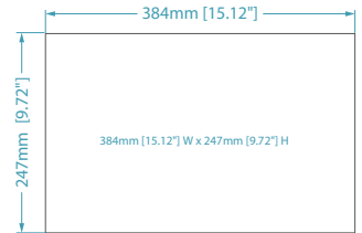
開孔尺寸
