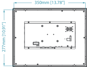
背視圖
