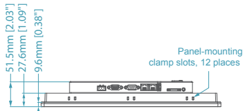
底視圖
