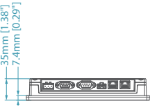
底視圖
