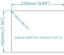
開孔尺寸
