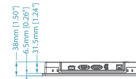
底視圖
