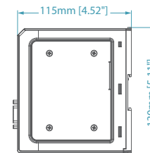
側視圖
