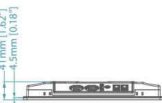
底視圖
