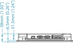
底視圖
