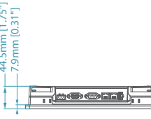
底視圖
