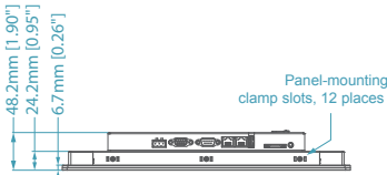
底視圖
