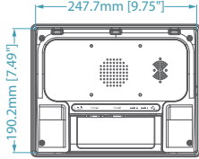
背視圖
