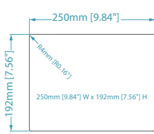
開孔尺寸
