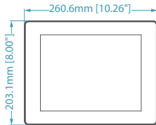
正視圖
