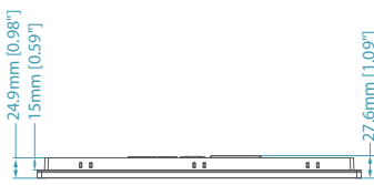
底視圖
