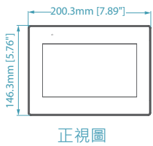
正視圖
