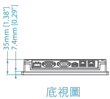
底視圖
