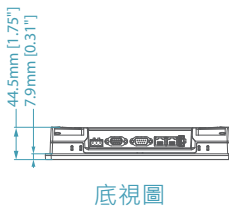
底視圖
