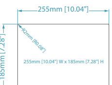
開孔尺寸
