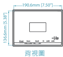
背視圖
