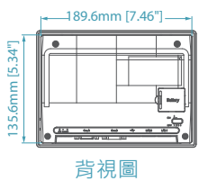
背視圖
