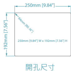
開孔尺寸
