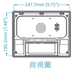
背視圖
