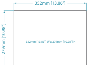
開孔尺寸
