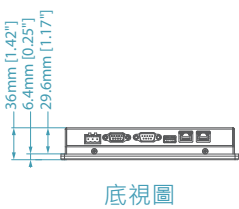
底視圖
