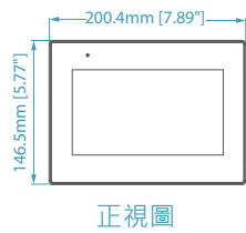
正視圖
