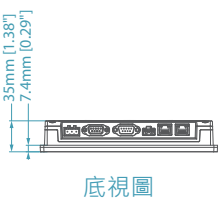
底視圖
