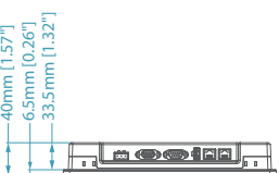
底視圖
