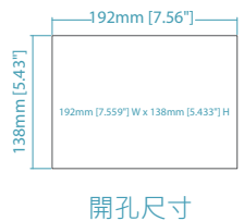
開孔尺寸
