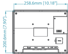
背視圖
