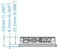
底視圖
