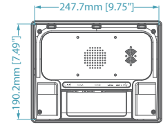
背視圖
