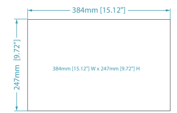
開孔尺寸
