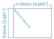
開孔尺寸
