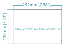
開孔尺寸
