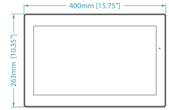
正視圖
