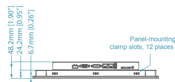
底視圖
