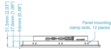
底視圖
