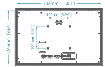
背視圖
