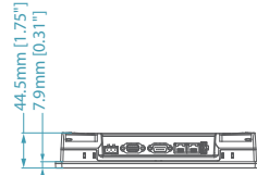
底視圖
