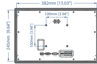
背視圖
