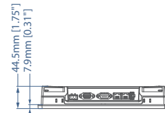
底視圖
