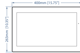
正視圖
