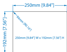
開孔尺寸
