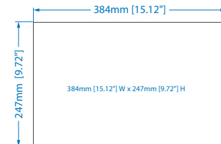
開孔尺寸
