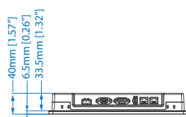
底視圖
