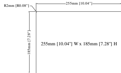
Cutout Dimensions
