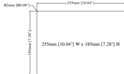
Cutout Dimensions
