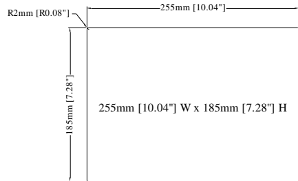
Cutout Dimensions
