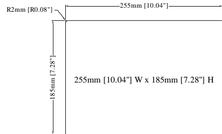
Cutout Dimensions
