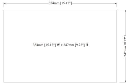
Cutout Dimensions
