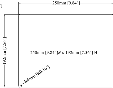
Cutout Dimensions
