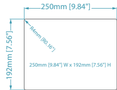
Cutout Dimensions
