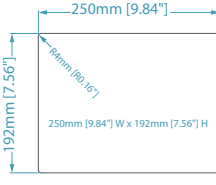
Cutout Dimensions
