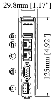
正面図
