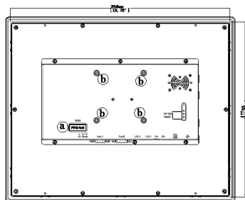
背面図
