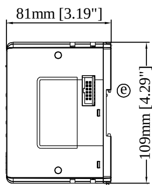
側面図
