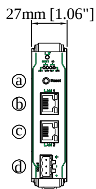
正面図
